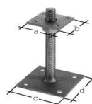
Pfostenträger höhenverstellb., verz. Art.-Nr. 218102 / GAH Platten zum Aufdübeln Preis: Fr. 29.00
