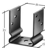
U-Pfostenlasche, verzinkt Zum Aufschrauben (ohne Schrauben) Art.-Nr. 217600 / GAH Für Pfosten 71/71 mm Preis: Fr. 8.00
