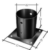
Aufschraubhülsen für Rundholz- pfosten verzinkt Art.-Nr. 211707 / GAH Durchmesser: 100 mm Preis: Fr. 17.00
