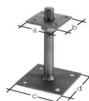
Pfostenträger höhenverstellb., verz. Art.-Nr. 218102 / GAH Platten zum Aufdübeln Preis: Fr. 28.00
