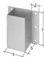
Pfostenträger, verzinkt zum Aufdübeln Art.-Nr. 208721 / GAH für Pfosten 70/70 mm Preis: Fr. 21.00
